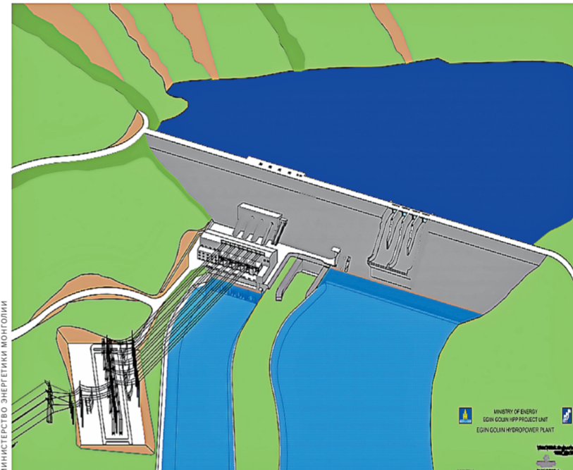
Красиво выглядит на картинке комплексный проект ГЭС «Эгийн-Гол» мощностью 315 МВт с годовой выработкой 606 ГВт/ч. Плотина ГЭС с рыбопропускным сооружением высотой 103 метра поднимется на 913 метров над уровнем моря. Этот проект тоже находится в пакете обсуждения.
