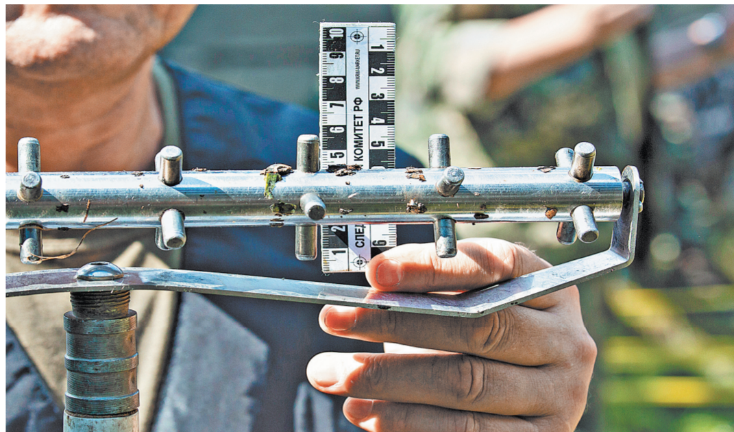
С помощью такого электромагнитного трапа криминалисты могут обнаружить под водой пули, гильзы и оружие.
